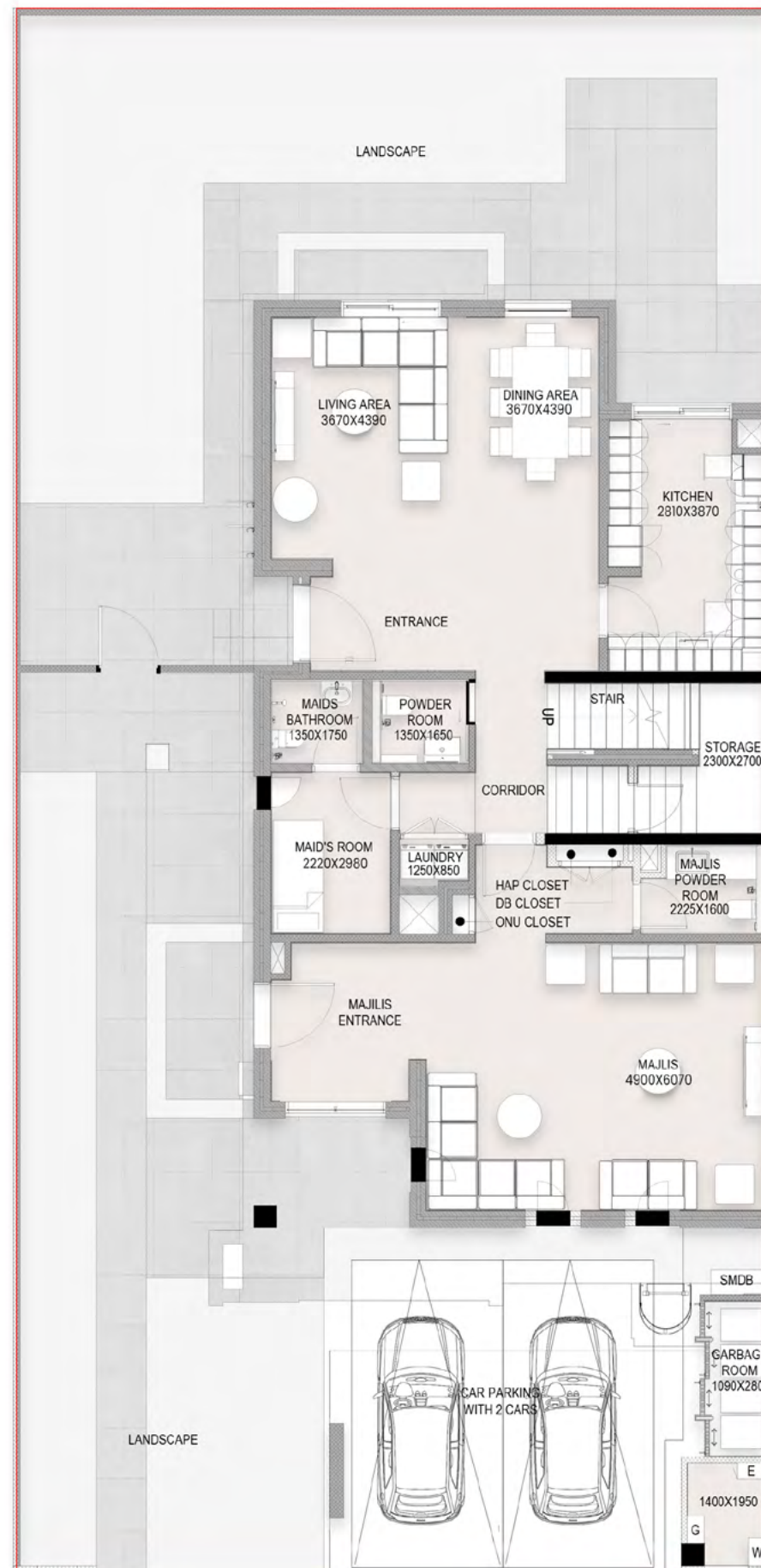
الطابق الأرضي 143.1 متر مربع
