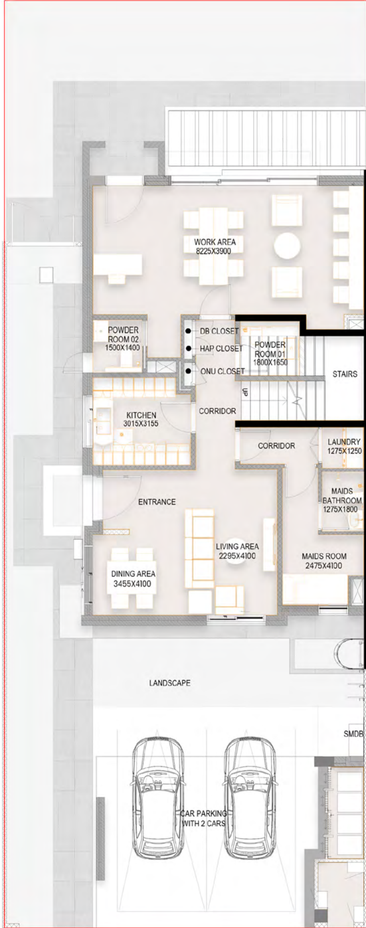
الطابق الأرضي 119.4 متر مربع
